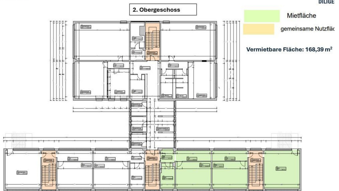
Grundriss- 2. OG
