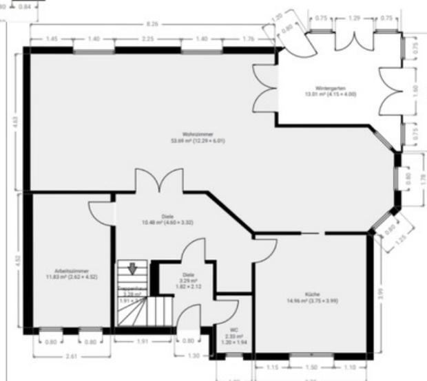
Grundriss EG mit Wintergarten
