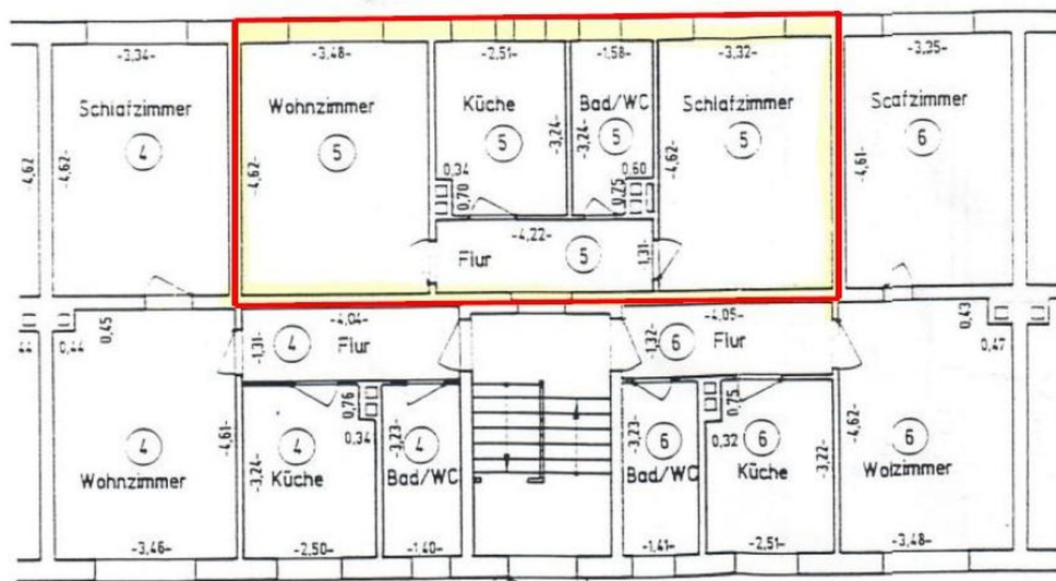
Grundriss Wohnung
