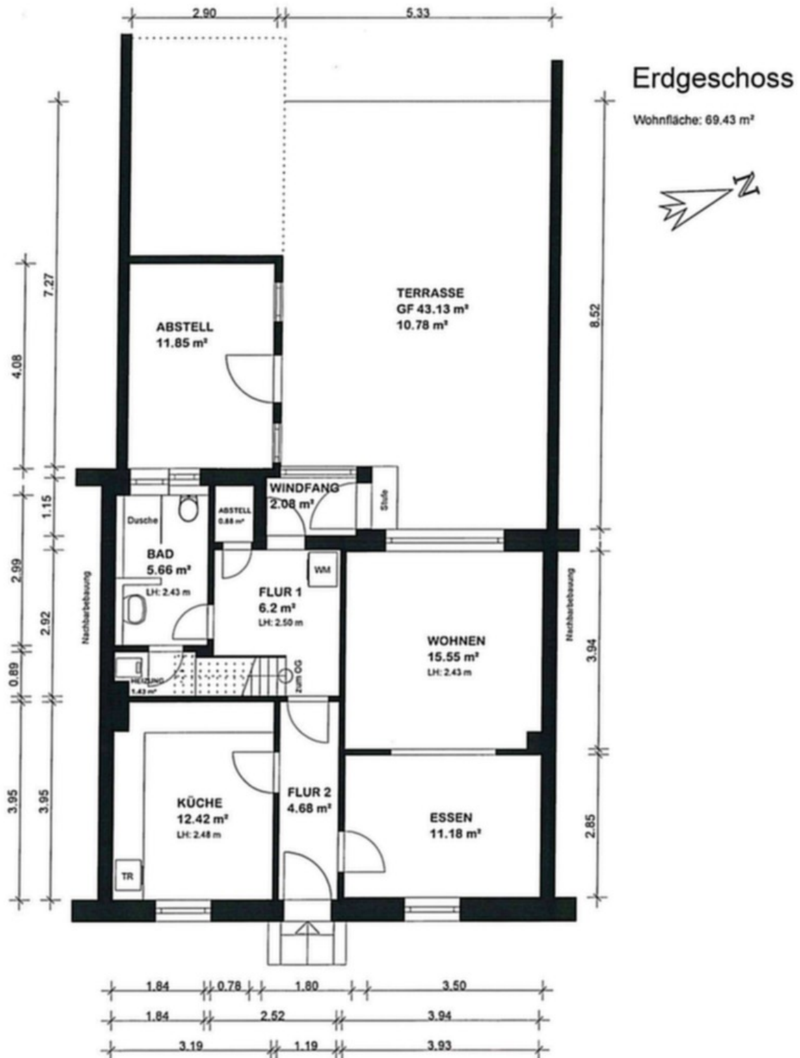
Grundriss EG
