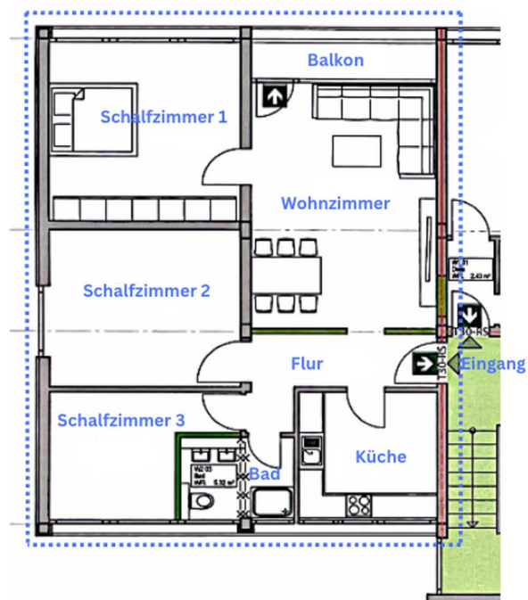
Grundriss
