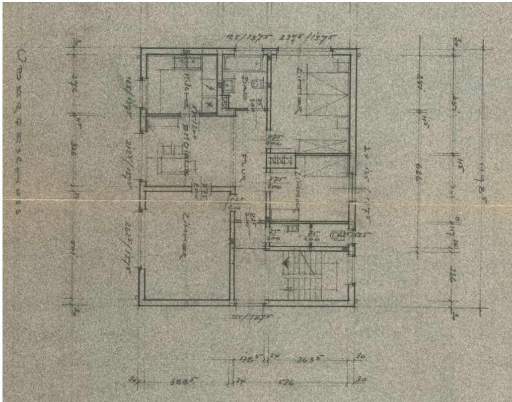
Grundriss des 1. OG
