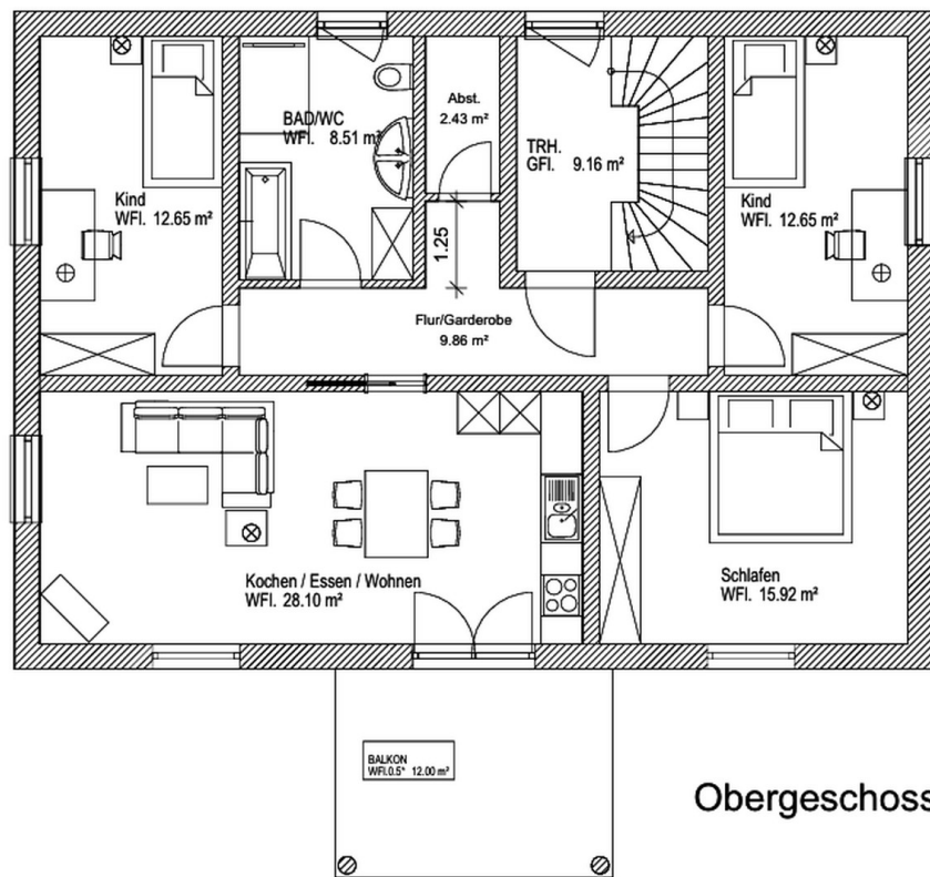
Grundriss_OG
