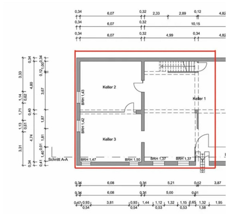
Grundriss Lagerkeller
