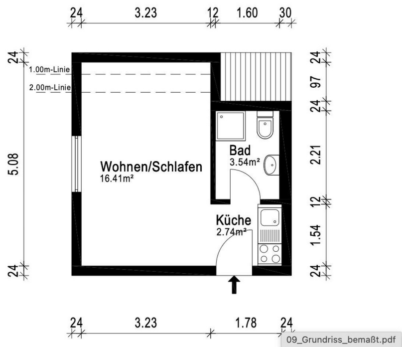
Grundriss
