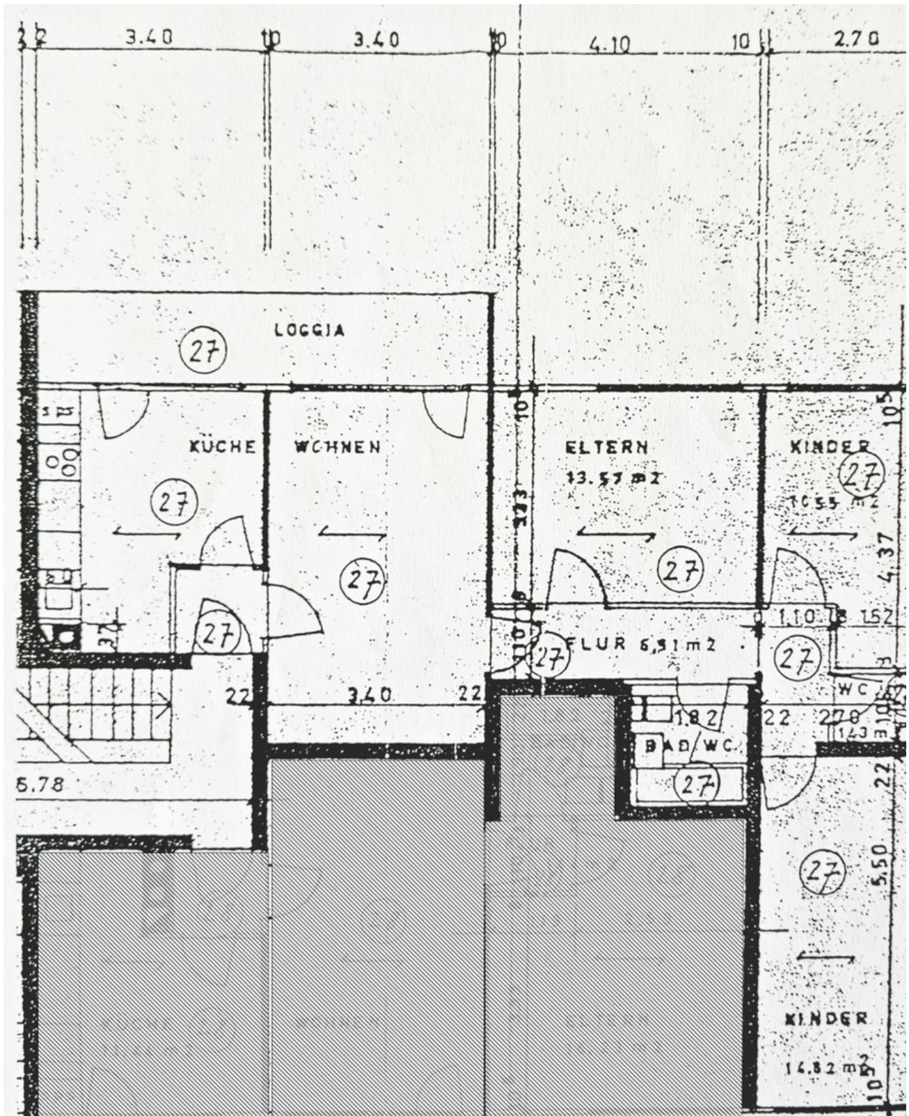
Grundriss Wohnung 27
