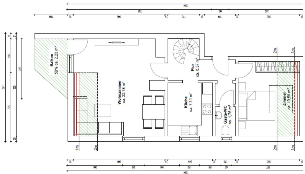
1.OG Grundriss
