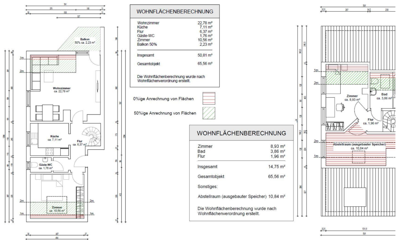
Grundriss - 2 Etagen
