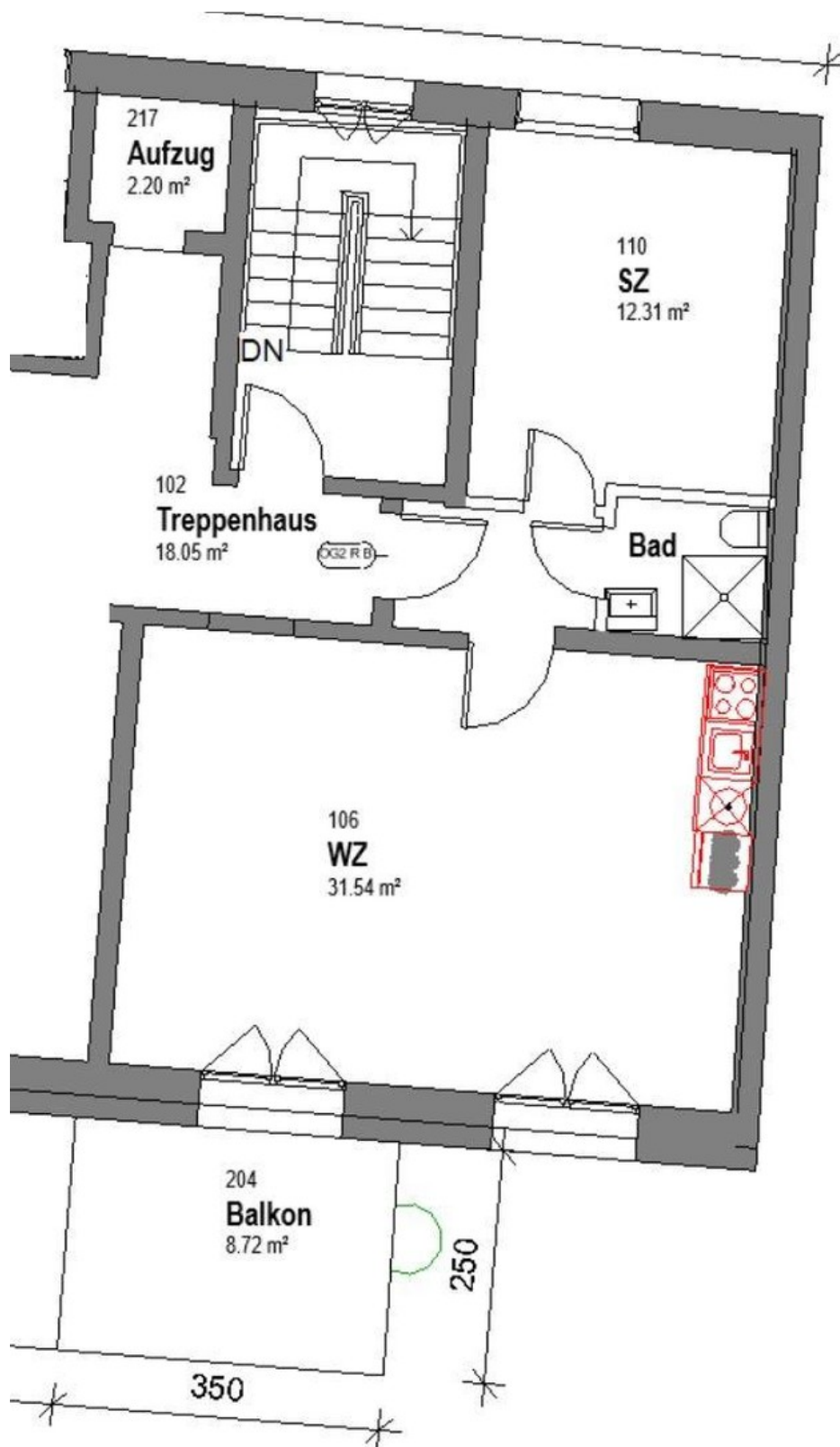
Grundriss
