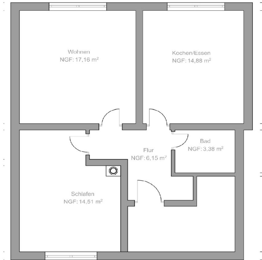
GRUNDRISS EG
