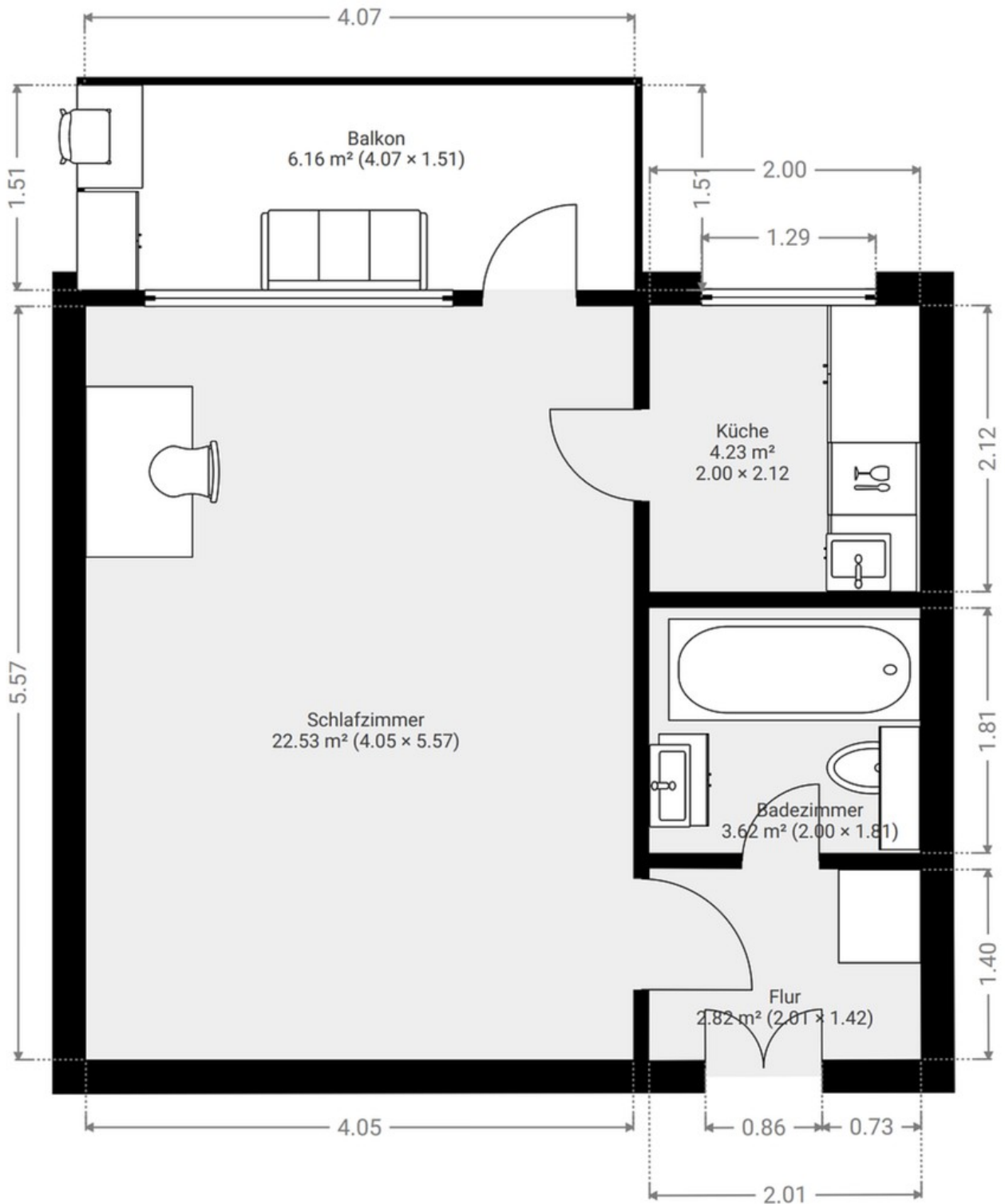
Grundriss
