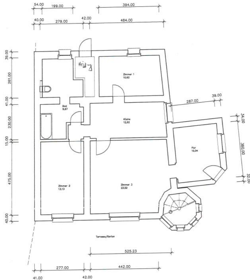
Erdgeschoss
