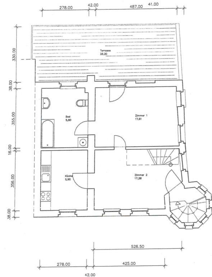
Obergeschoss
