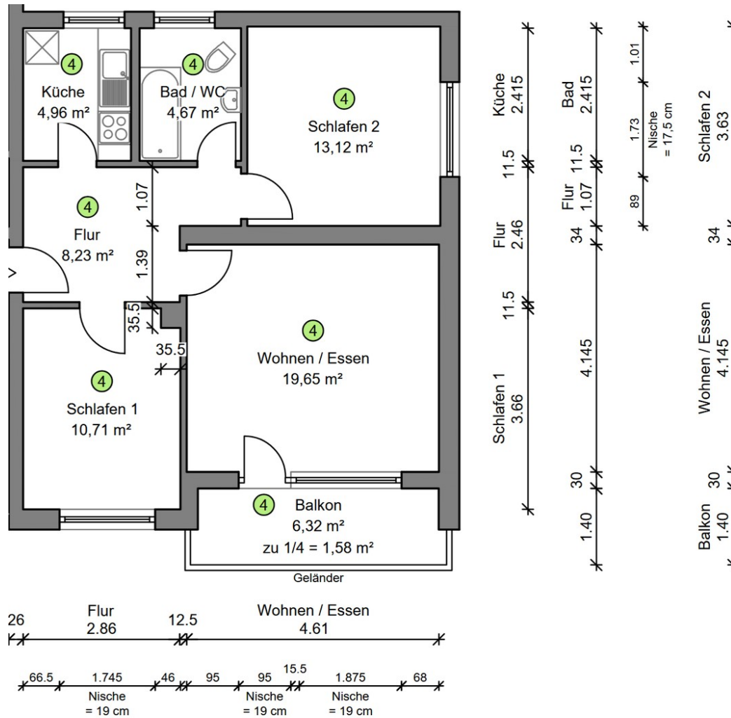
Grundriss I. OG rechts
