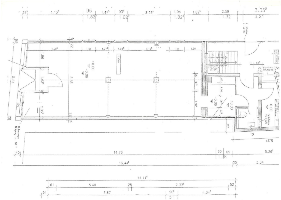
Grundriss Ladenlokal
