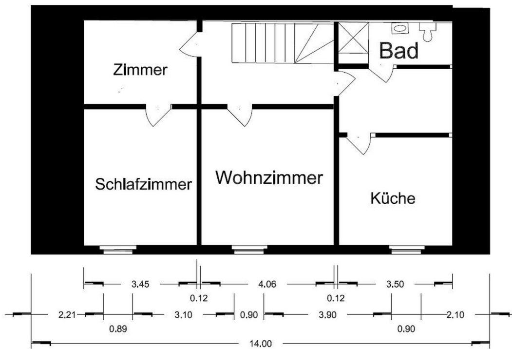
2. Obergeschoss
