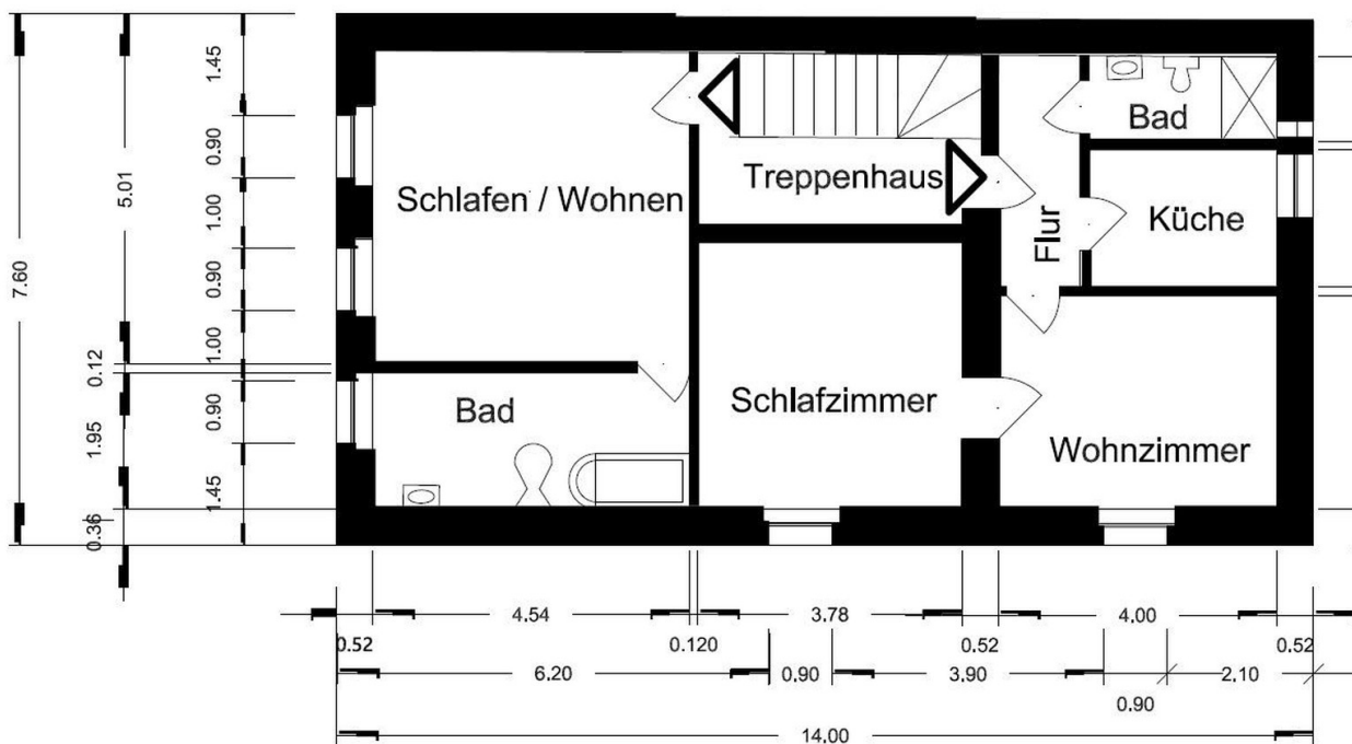
1. Obergeschoss
