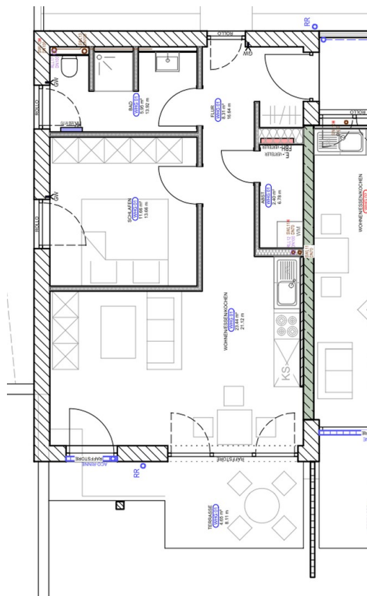
Grundrissplan
