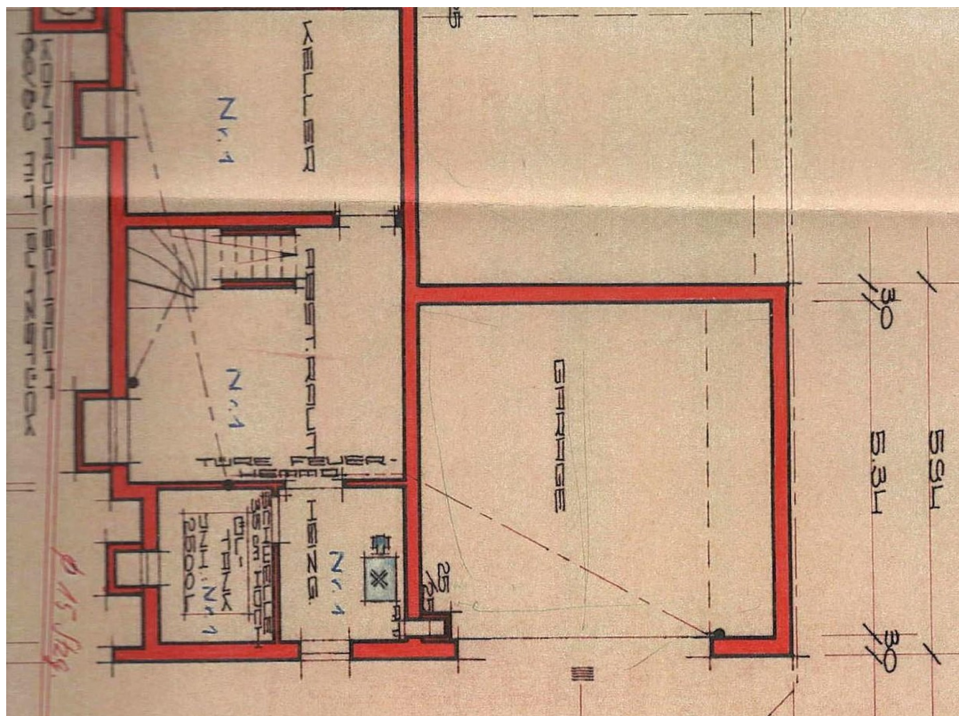
Grundriss UG
