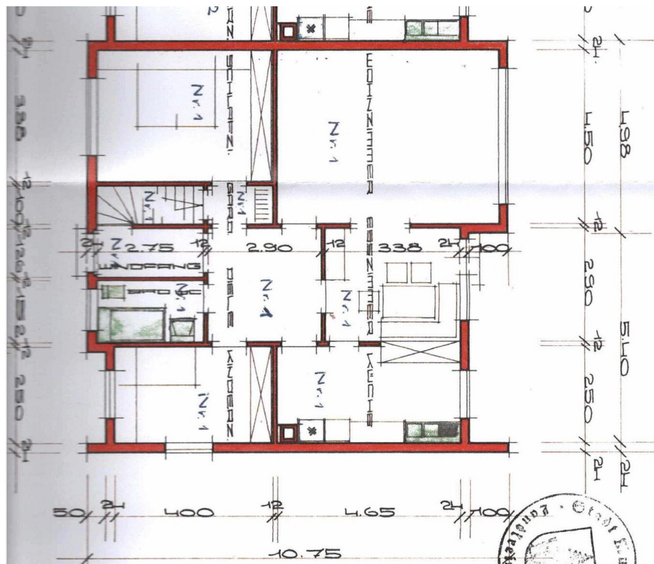
Grundriss EG
