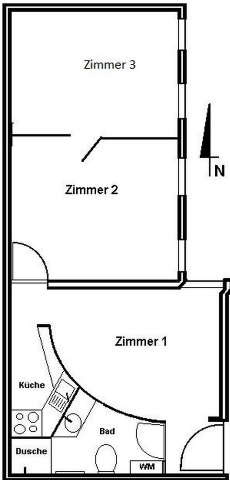
Grundriss Erdgeschoss
