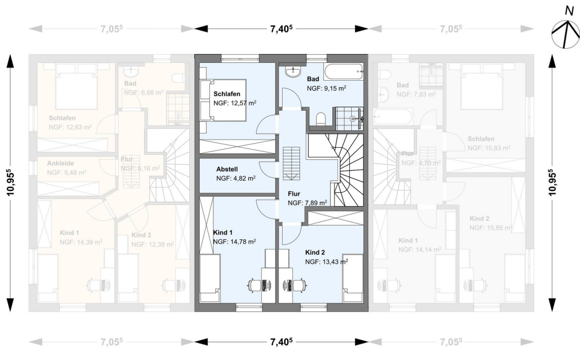
Grundriss Obergeschoss
