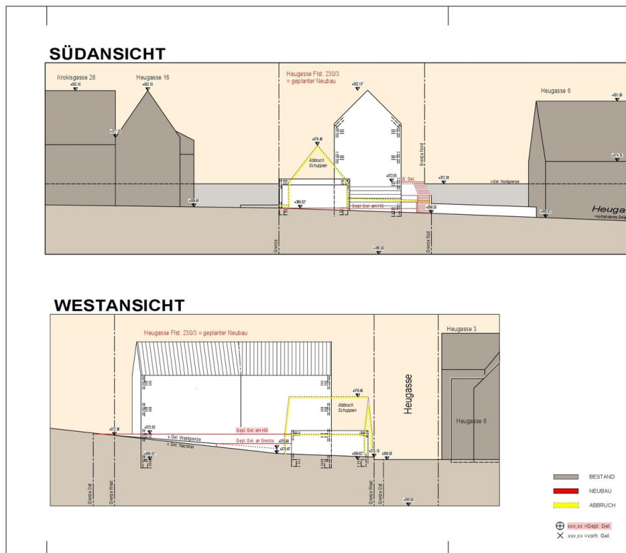
Süd + Westansicht
