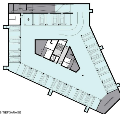
GRUNDRISS TIEFGARAGE
