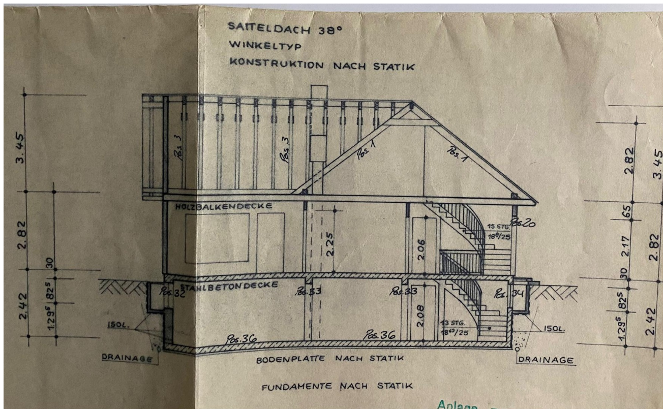
Querschnitt Haus
