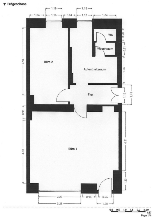
Derzeitiger Grundriss
