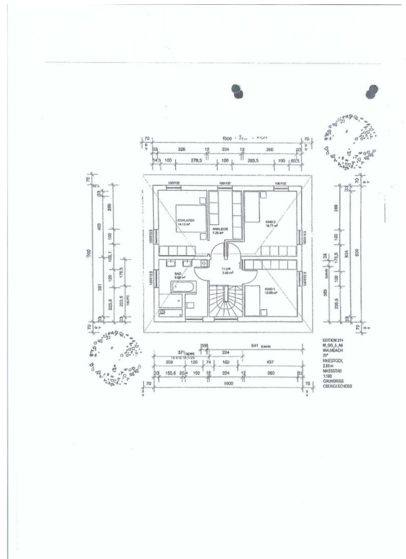
Grundriss OG
