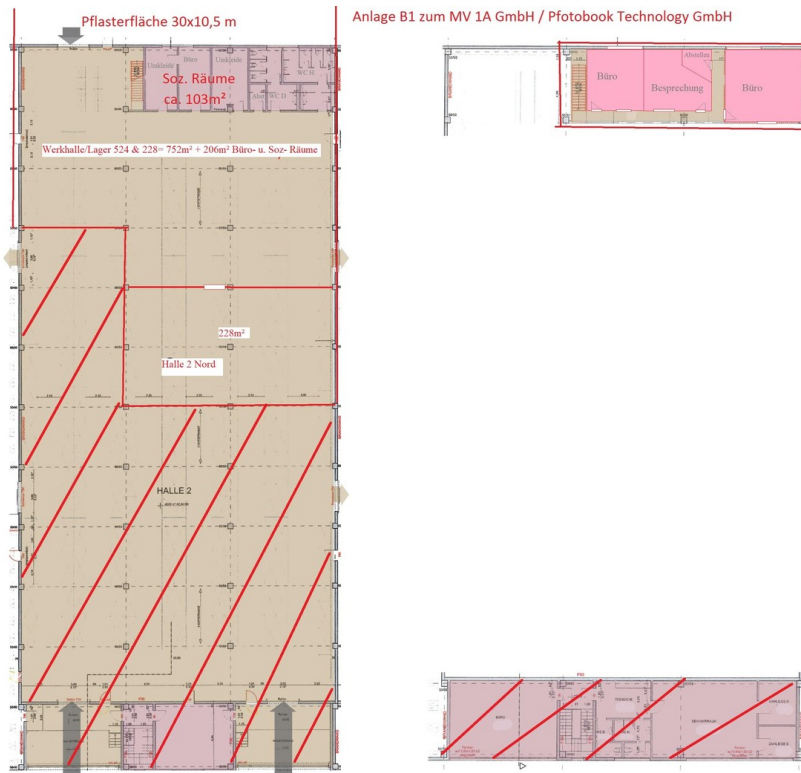
Grundriss
