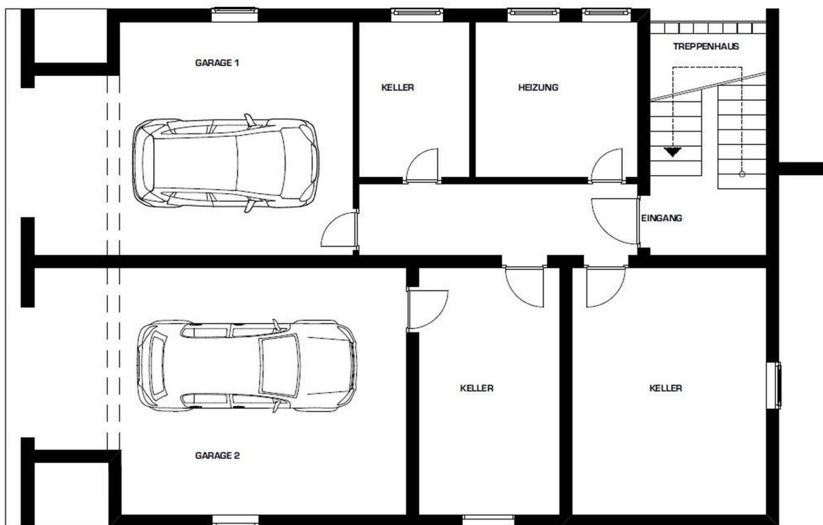
Grundriss KG
