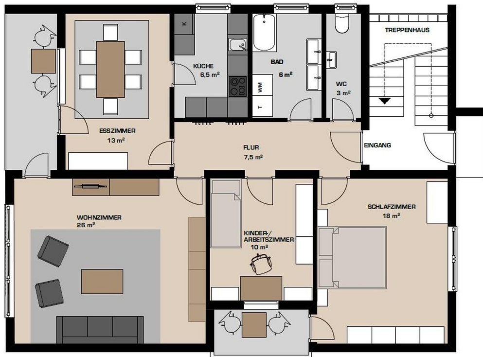
Grundriss 1. OG
