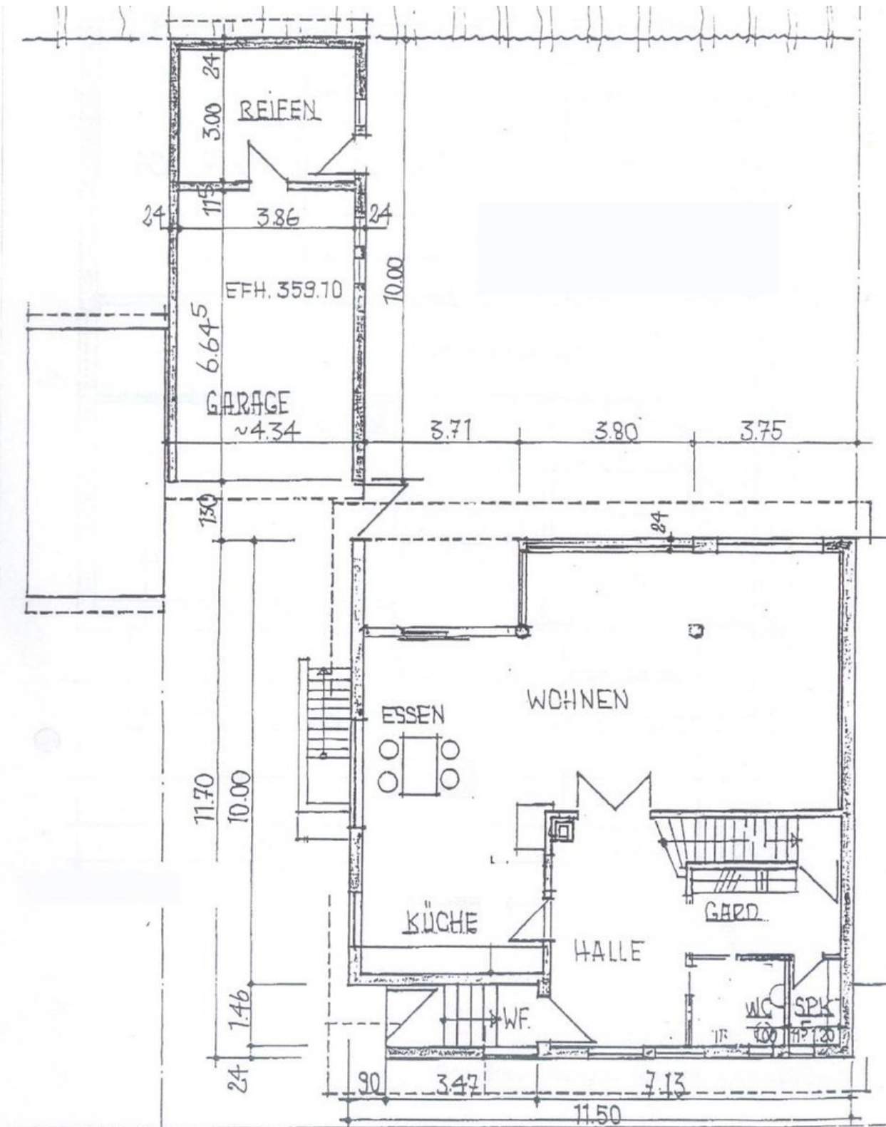
Grundriss EG
