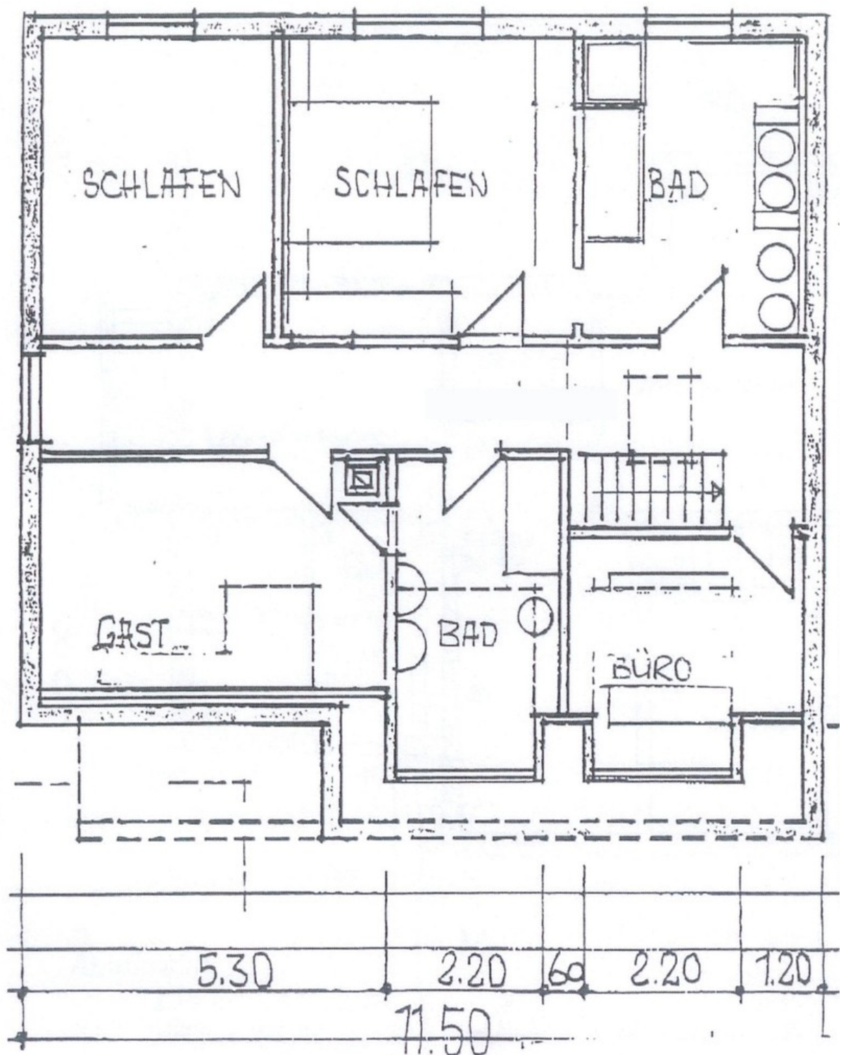
Grundriss OG
