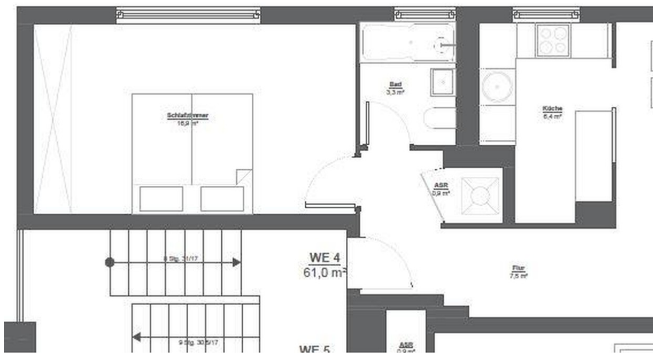
Grundriss
