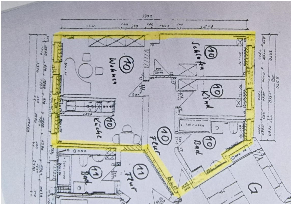
Grundriss Wohnung
