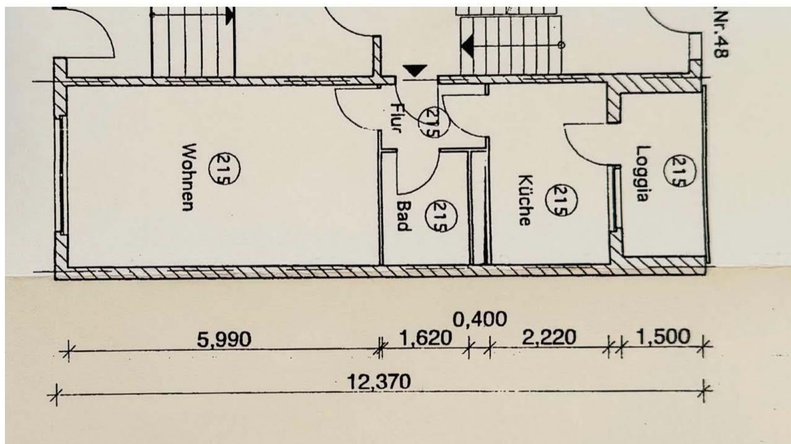
Grundriss Wohnung
