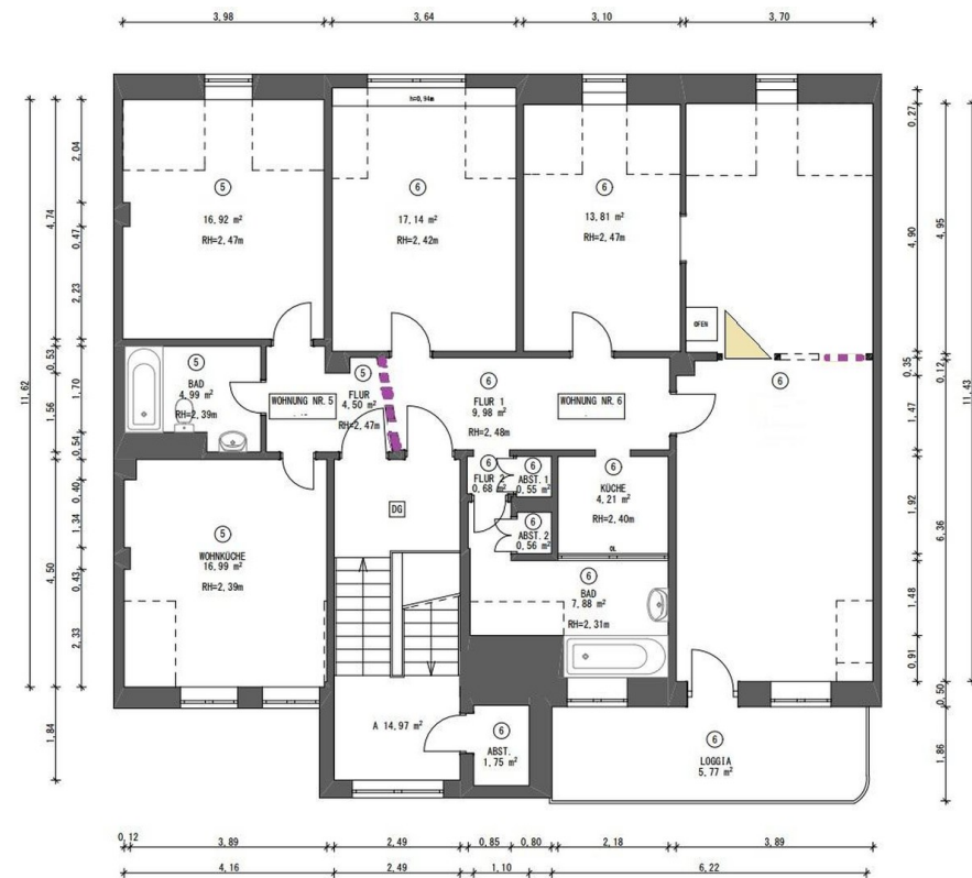
Grundriss bei Zusammenlegung
