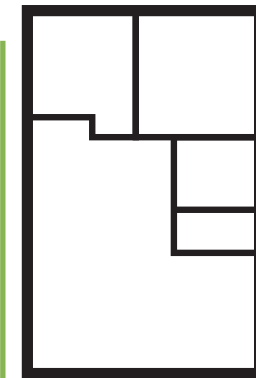
WOHNUNG 7 Wohnfläche: 51,11 Balkon: - Gesamt: 51,11
