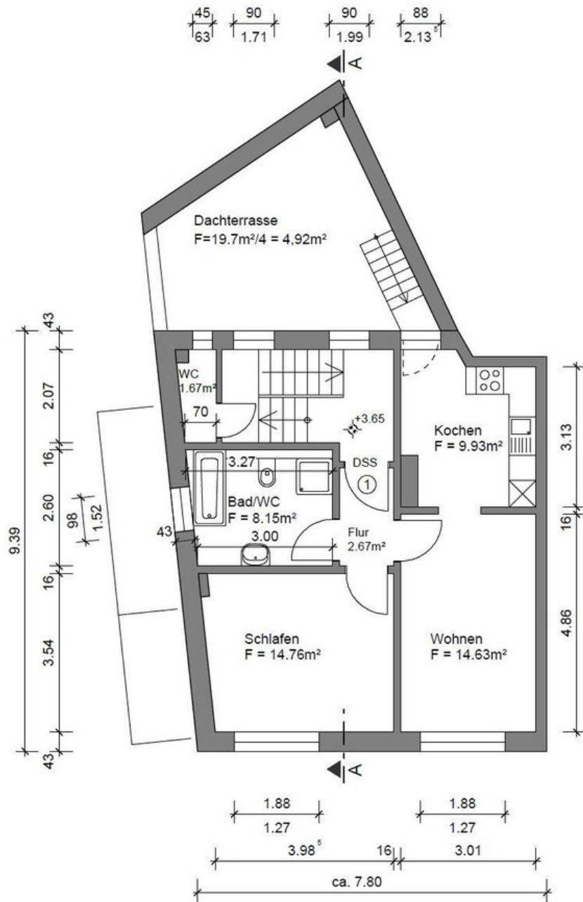
1. OBERGESCHOSS
