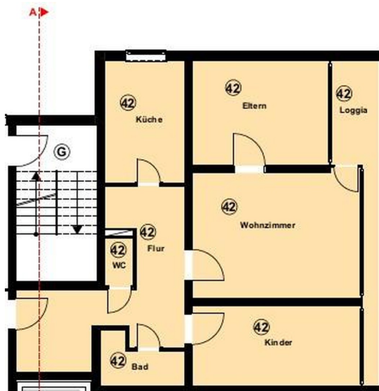
Grundriss
