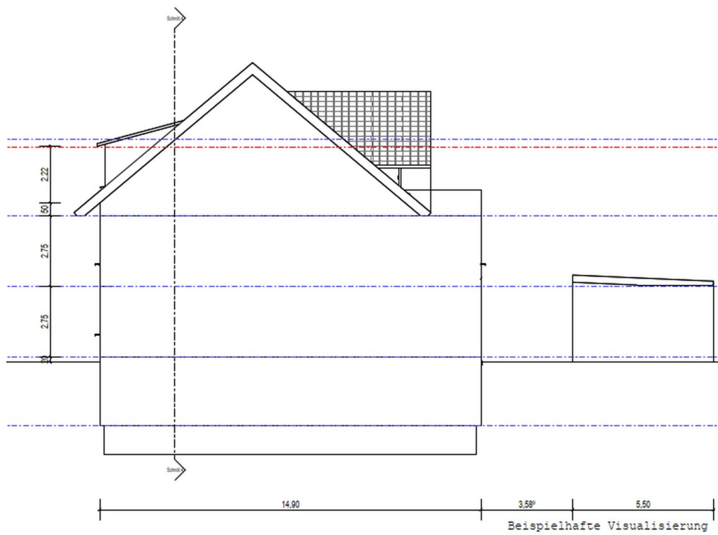
Geplante Ostansicht
