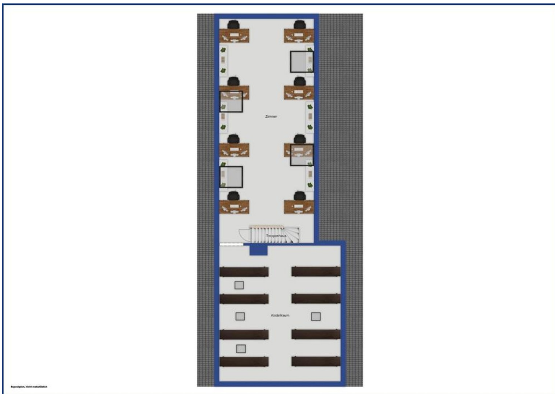
Grundriss Dachgeschoss
