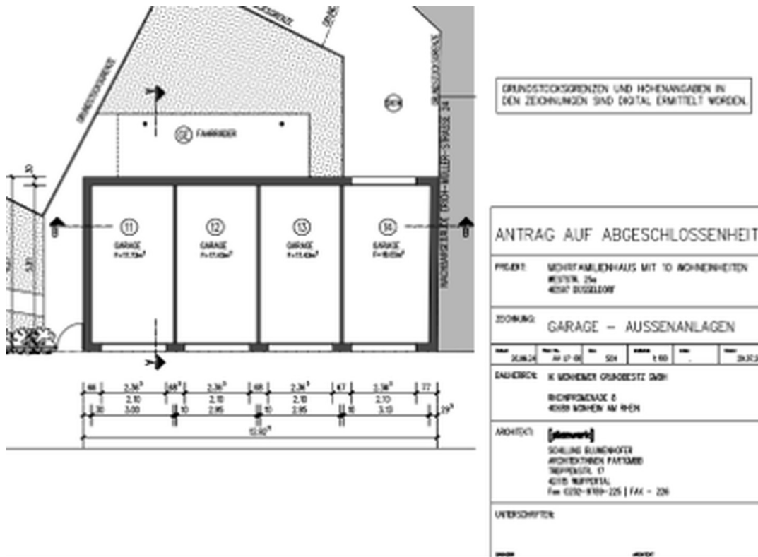
Grundriss
