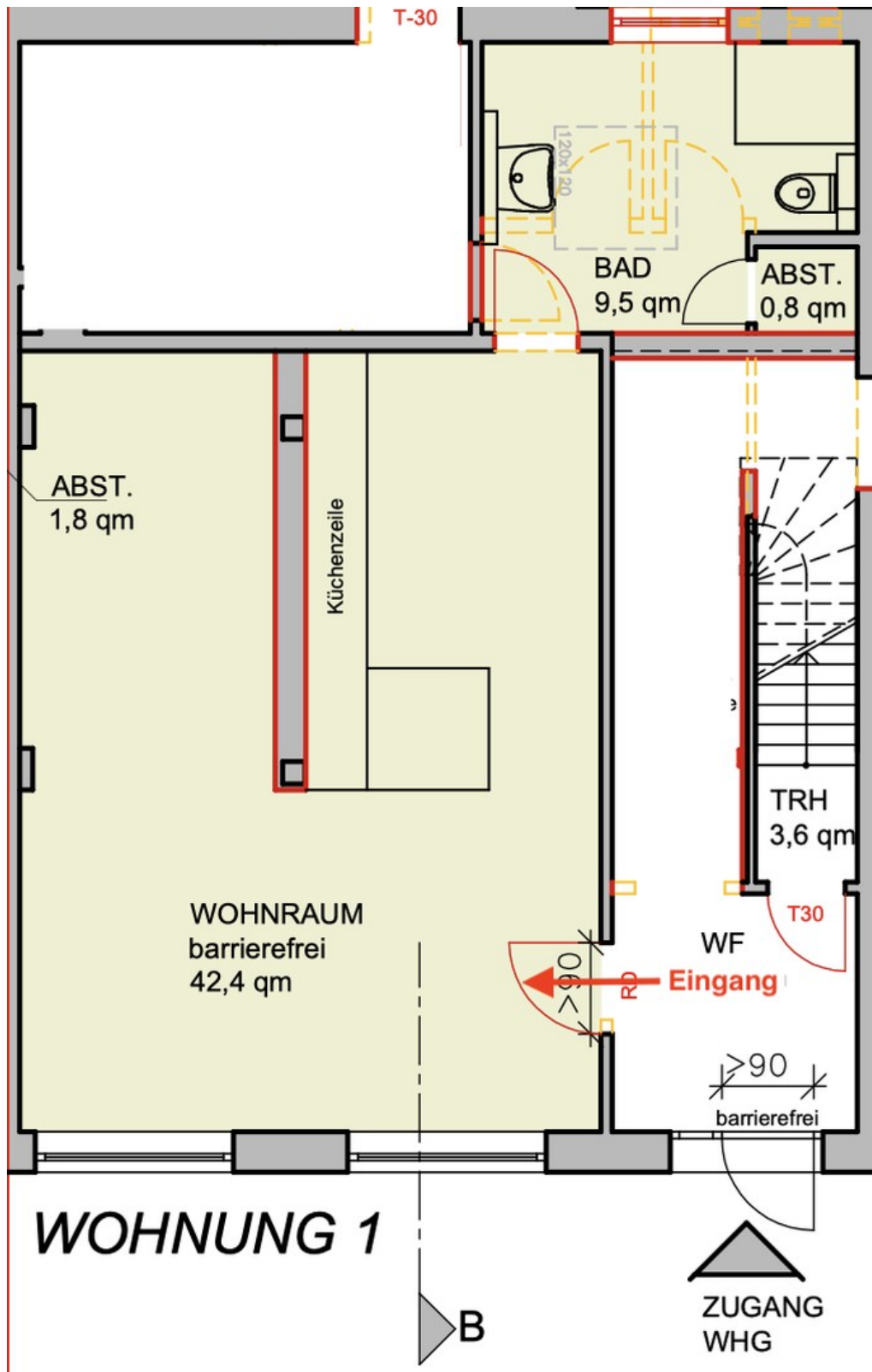
Grundriss
