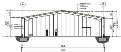
Schnitt 1-1
