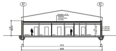
Schnitt 2-2
