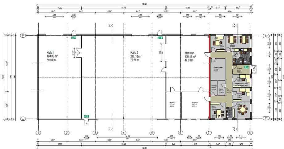
Grundriss
