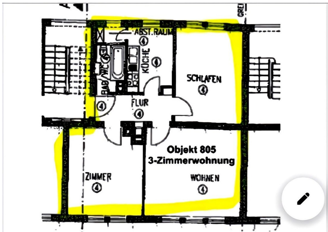
Grundriss
