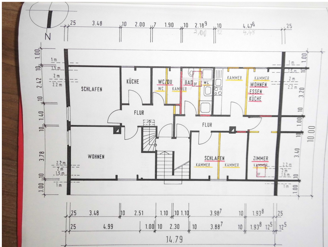
Dachstockumbau 1994
