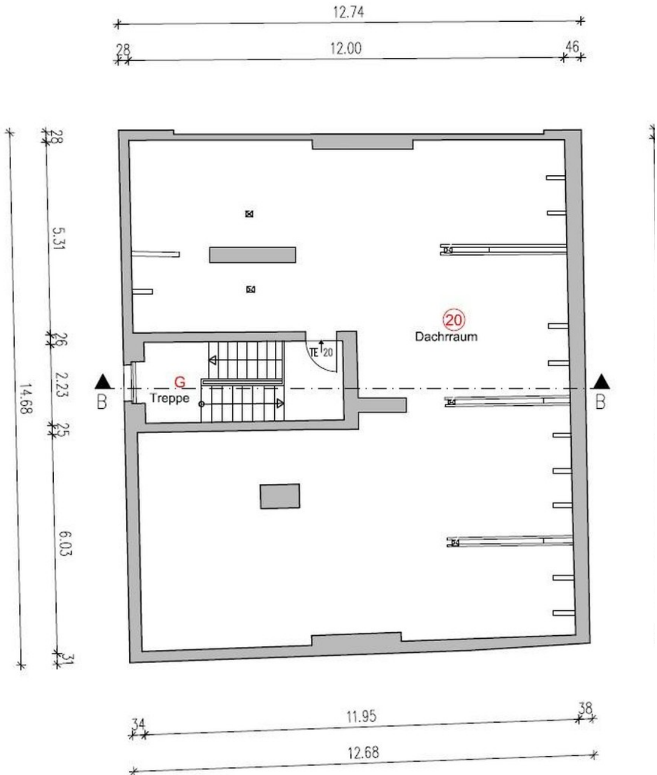
Grundriss Dach
