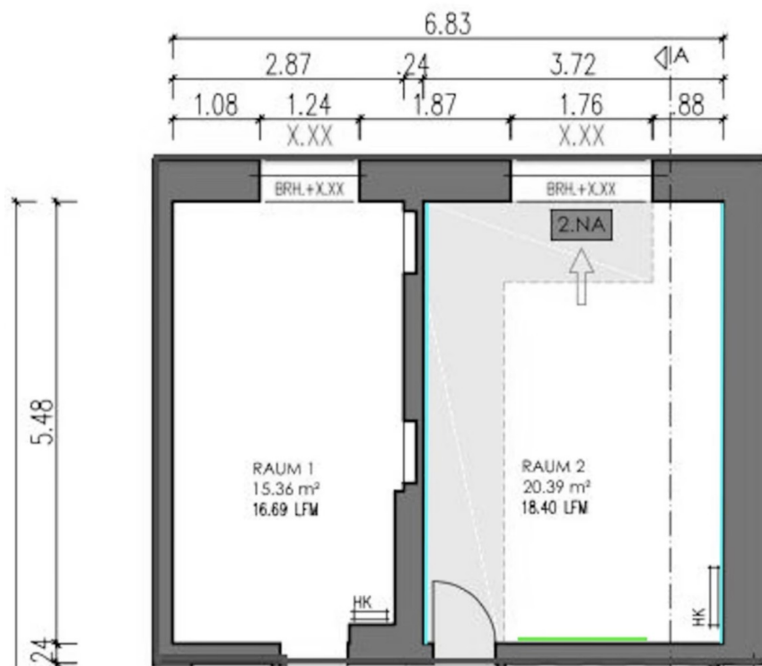
Grundriss plus WC
