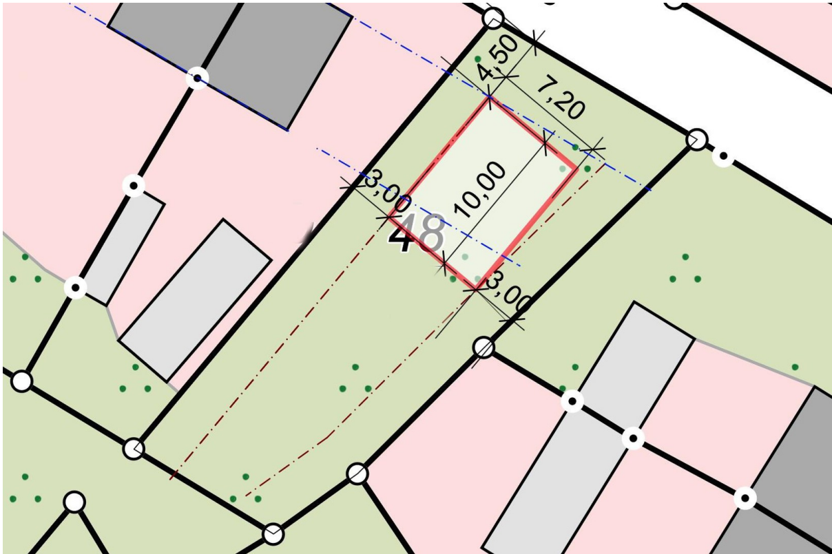
Skizze Grundfläche Bebauung
