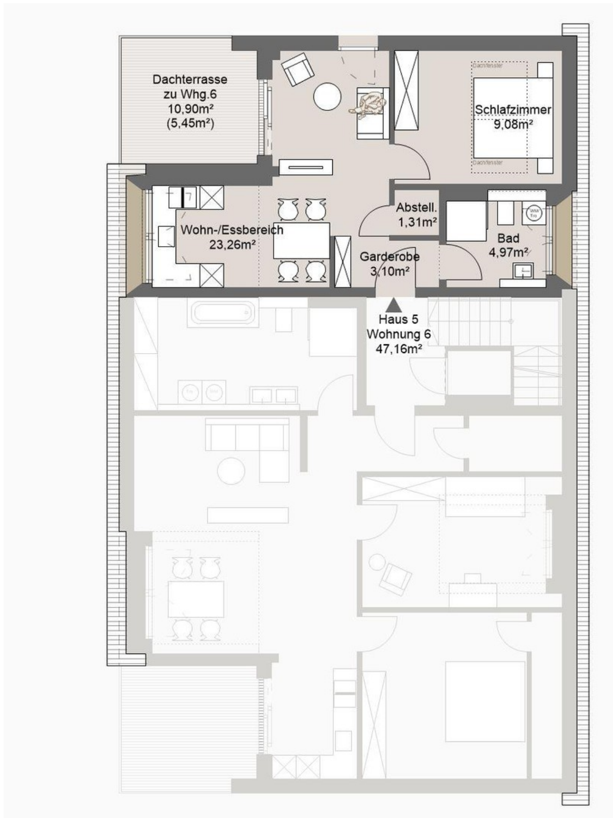
Wohnung 6 im DG
