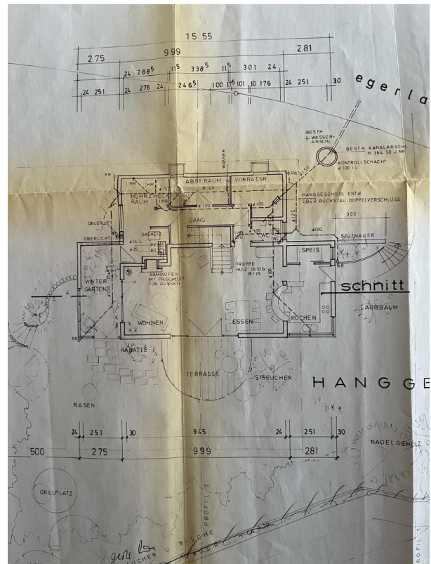
Grundriss Parterre
