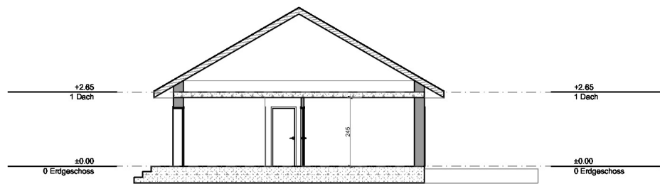
Schnitt 1:100
